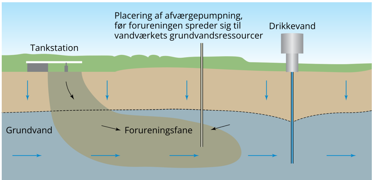
Fig. 5.13: Principskitse af forureningsoprensning ved en afværgepumpning. (Illustration: Jørgen Strange).
